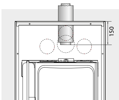
Aspirazione/Scarico coassiale 60/100 verticale
