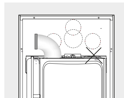
Aspirazione/Scarico coassiale 60/100 laterale destro
